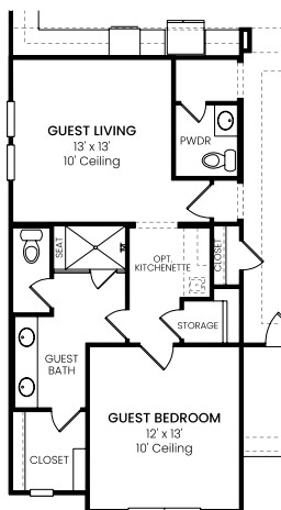
OPTIONAL GUEST SUITE
