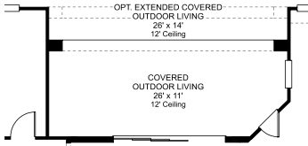
OPTIONAL 12' x 8' SLIDING GLASS DOOR
