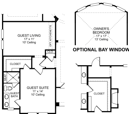
OPTIONAL GUEST SUITE
