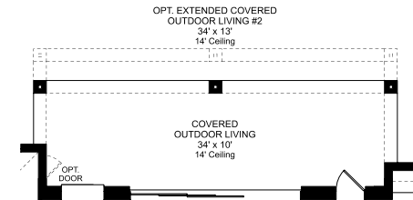
OPTIONAL 16' x 8' SLIDING GLASS DOOR
