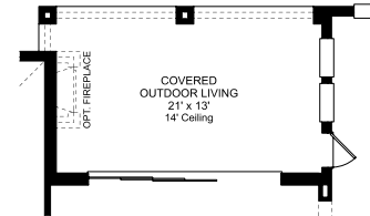
OPTIONAL 15' x 8' SLIDING GLASS DOOR
